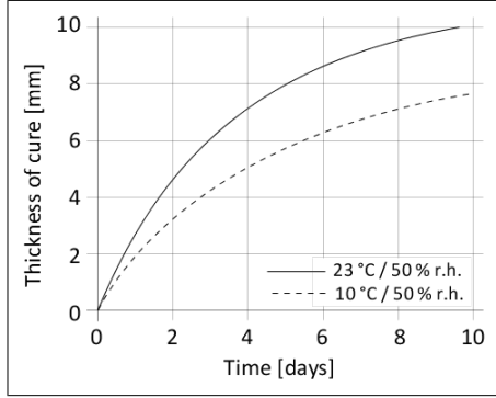
Biểu đồ 1: Tốc độ đóng rắn của Sikaflex®-515
