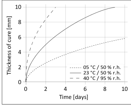
Biểu đồ 1: Tốc độ đóng rắn của Sikasil® WS-355 N
